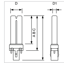
Philips PL-S 9W /12 G23
